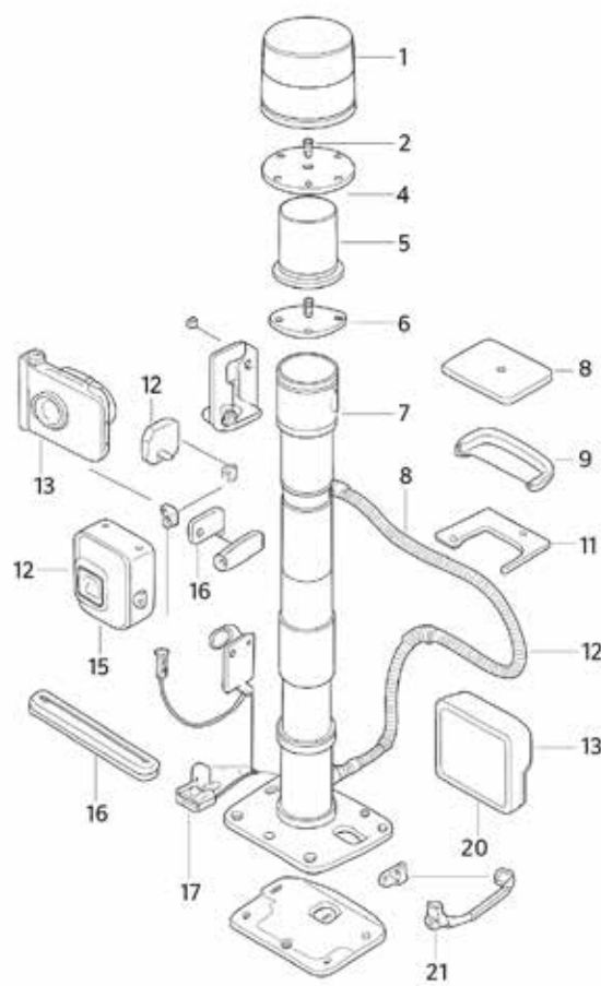
Onderdelen diagram
